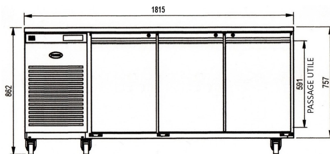
VUE DE FACADE
